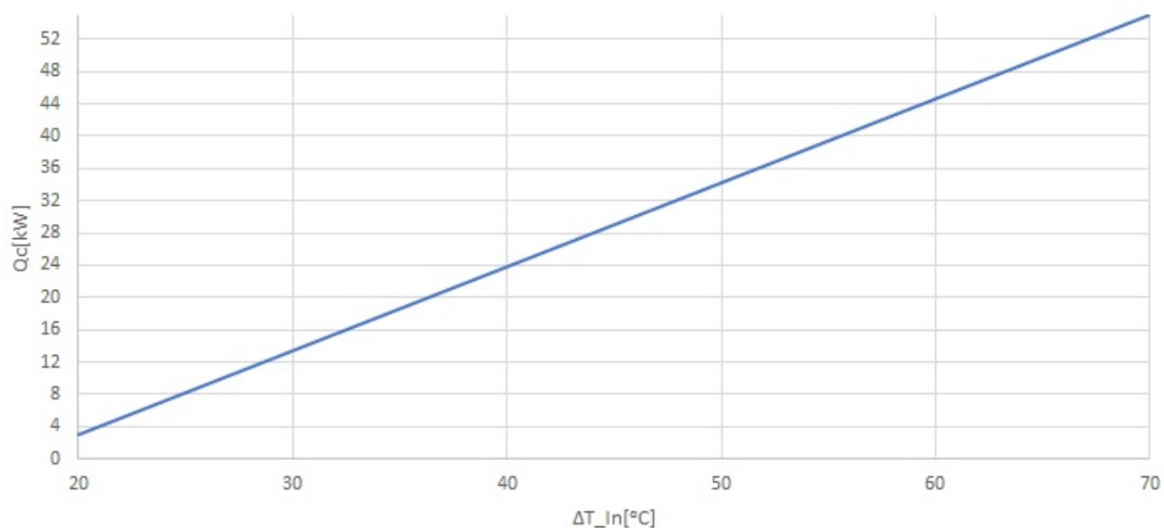
Moc nagrzewnicy (6 rzędowej) w funkcji średniej różnicy temperatury przy przepływie 600m 3 /h
