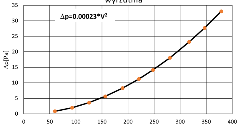
Charakterystyka hydrauliczna nawiewnik K3 wyrzutnia
