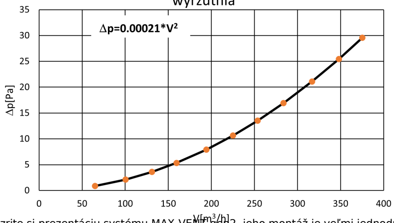
Charakterystyka hydrauliczna nawiewnik K5 wyrzutnia
