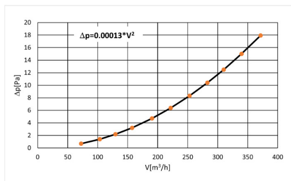
rys. 4. Charakteristika hydraulická výzuti K1.
