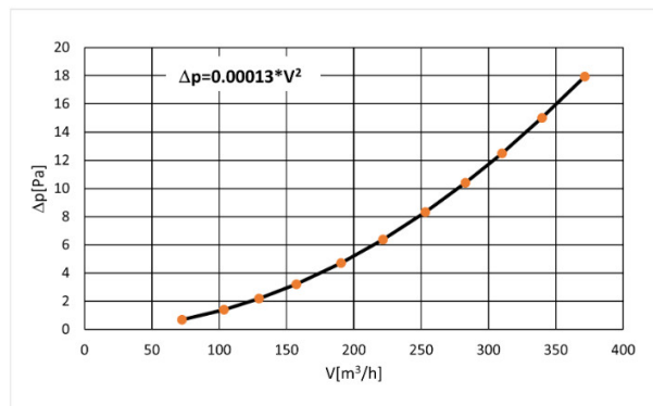
rys. 4. Charakteristika hydraulická výstupu K1.
