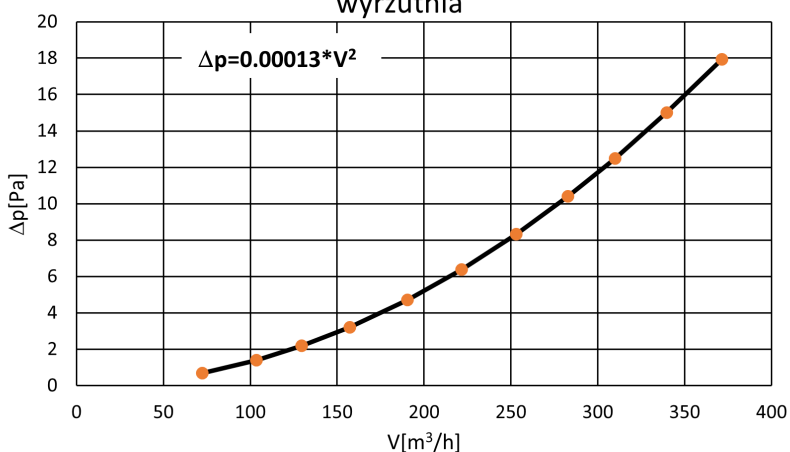
Charakterystyka hydrauliczna nawiewnik K1 wyrzutnia
