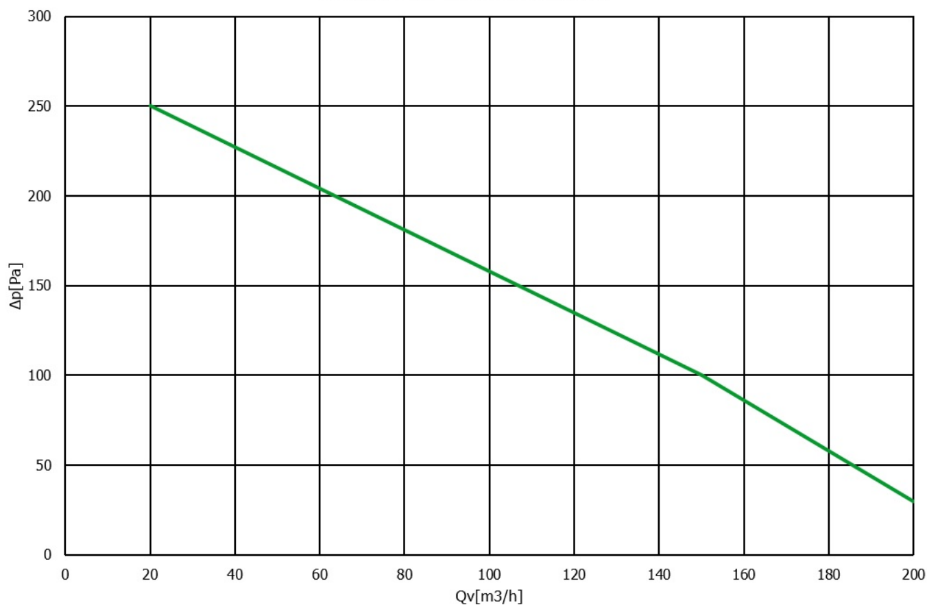
Sprež centrali w funkcji przepływu
